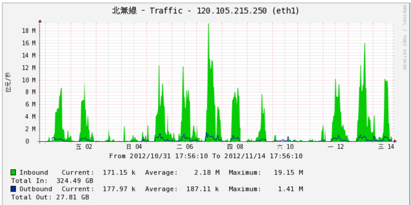
圖 3. 北無線網路伺服器兩星期網路流量圖
