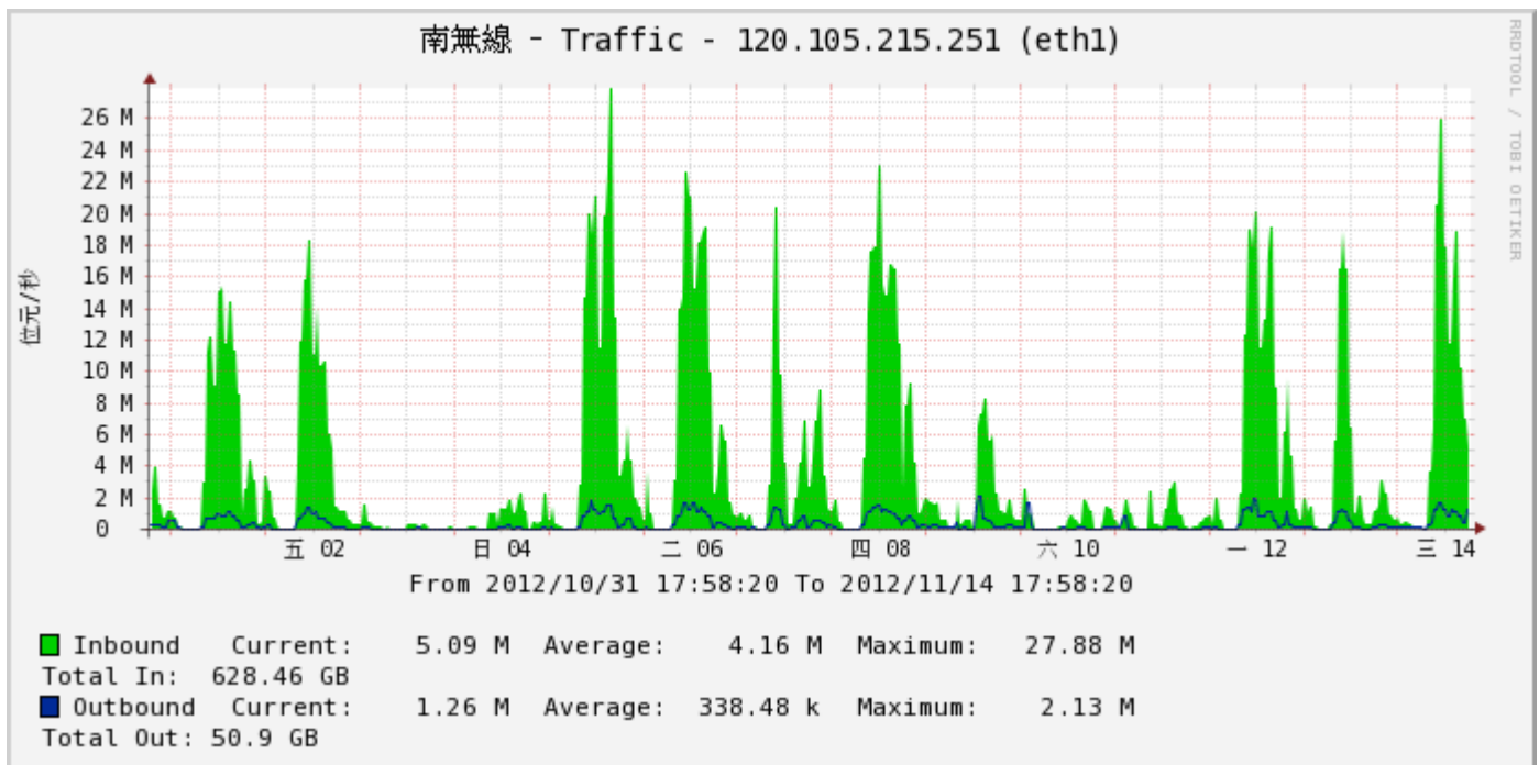
圖 4. 南無線網路伺服器兩星期網路流量圖
